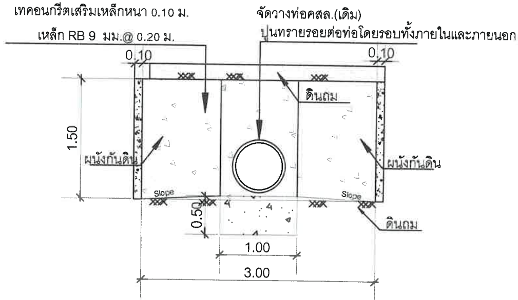
แบบรูปด้านแสดงการจัดวางท่อระบายน้ำ คสล. มาตราส่วน 1 : 50
