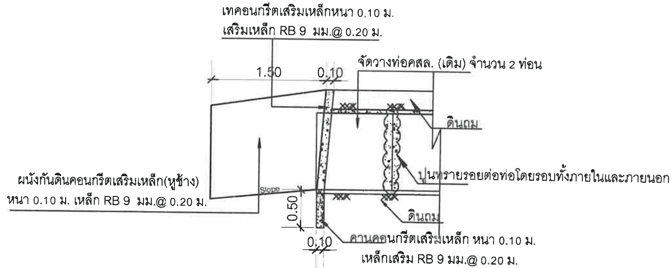
แบบรูปตัดแสดงพื้น / ผนังกันดิน คสล.(หูช้าง) มาตราส่วน 1 : 50
